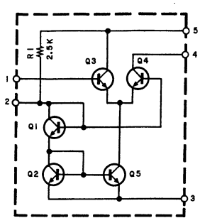
Fig. 7.1.7 FM IF Amp. IC TA7060AP
